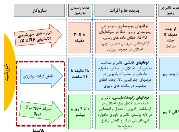
شکل ۱. سازوکار رخدادهای اقلیم فضا، مدت و نوع تاثیرات آنها بر سامانه‌های فضایی و زمینی
