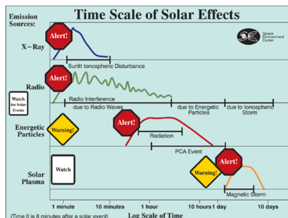
شکل ۳. فرصت‌ها و بازه‌های زمانی معمول برای اعلان خطر در صورت بروز رخدادهای اقلیم فضا [۱۰]
