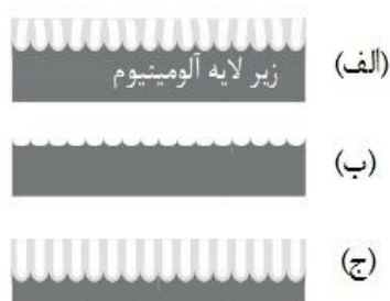
شکل ۲. مراحل فرایند ساخت الگوی اکسید آندی آلومینیوم
